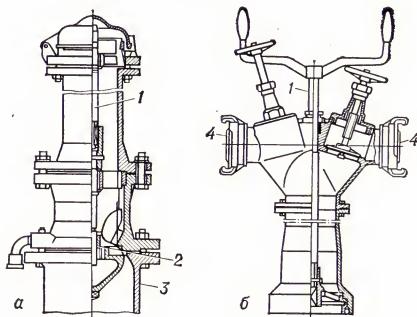
Гидрант-колонка (а) и подземный гидрант (б): 1 — штанга; 2 — клапан; 3 — пожарная подставка; 4 — напорный патрубок.
